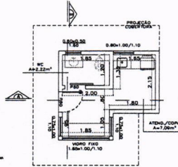
PLANTA BAIXA DE: VISO
