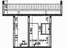
CORTE BB DE: VISO
