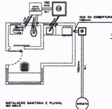
METALIZAÇÃO SANITÁRIA E PLUVIAL DE: VISO
